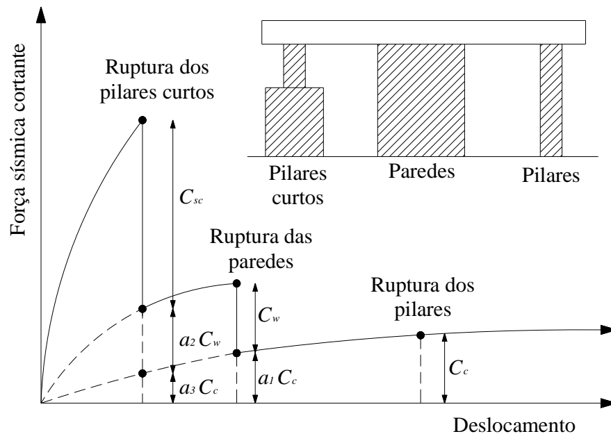
Figura 16 – Comportamento dos diferentes elementos verticais
