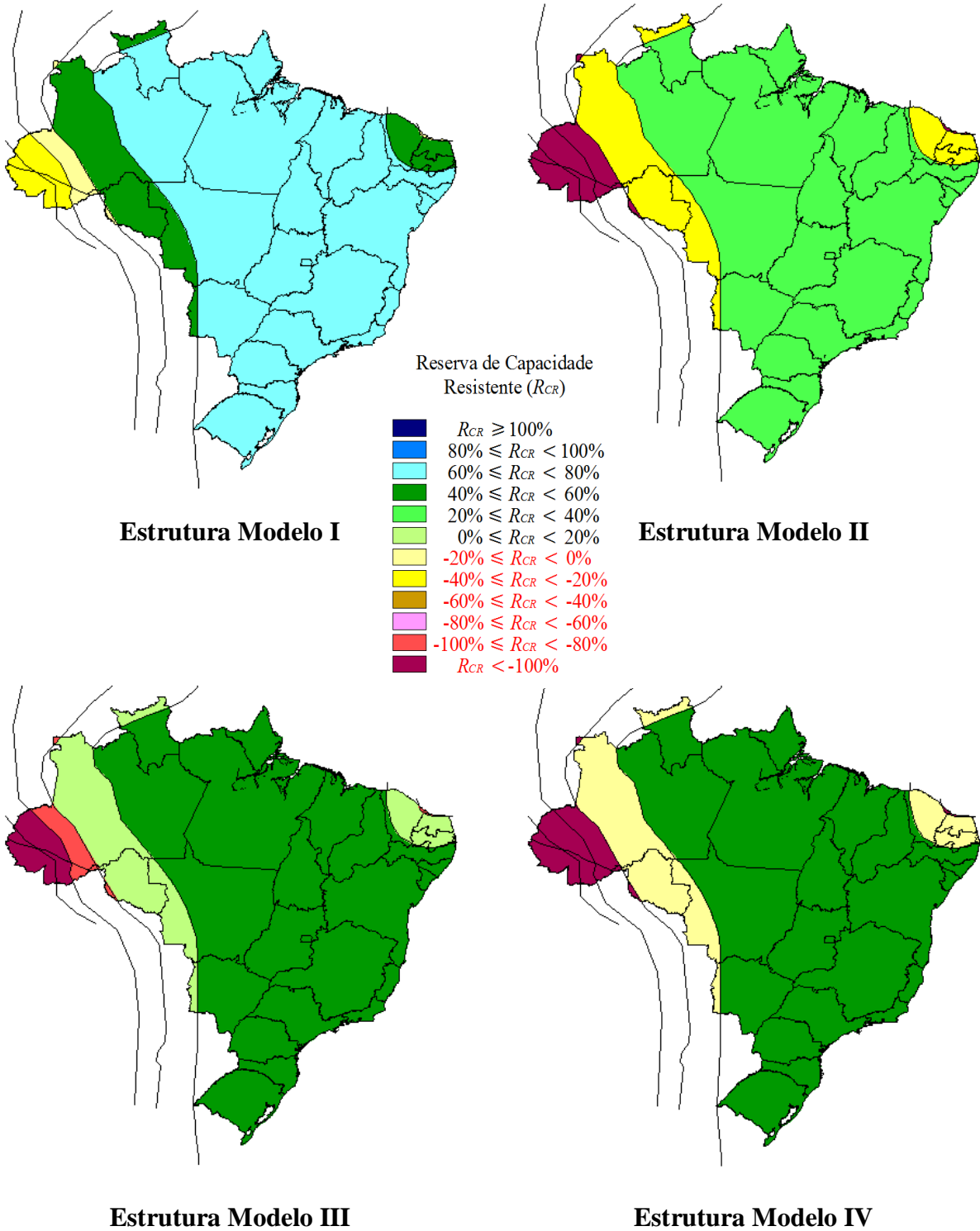
Figura 53 - Mapas de vulnerabilidade sísmica das estruturas modelo – Terreno Classe E
