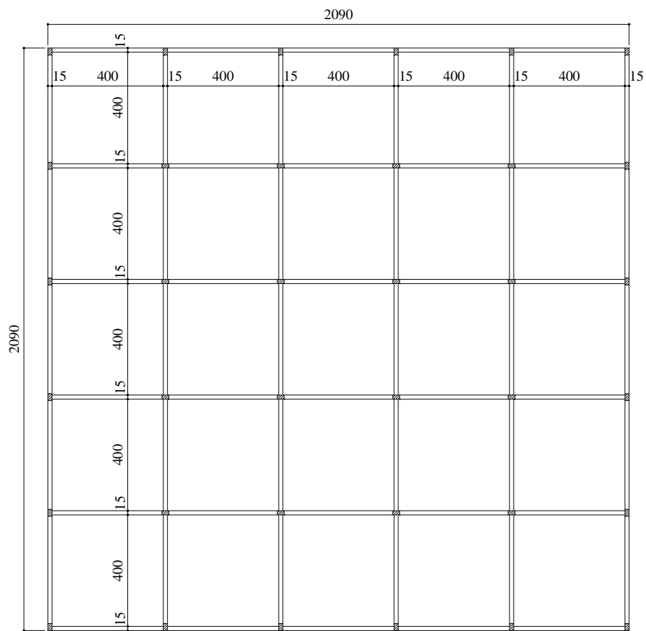
Forma do pavimento Nível +2,80
