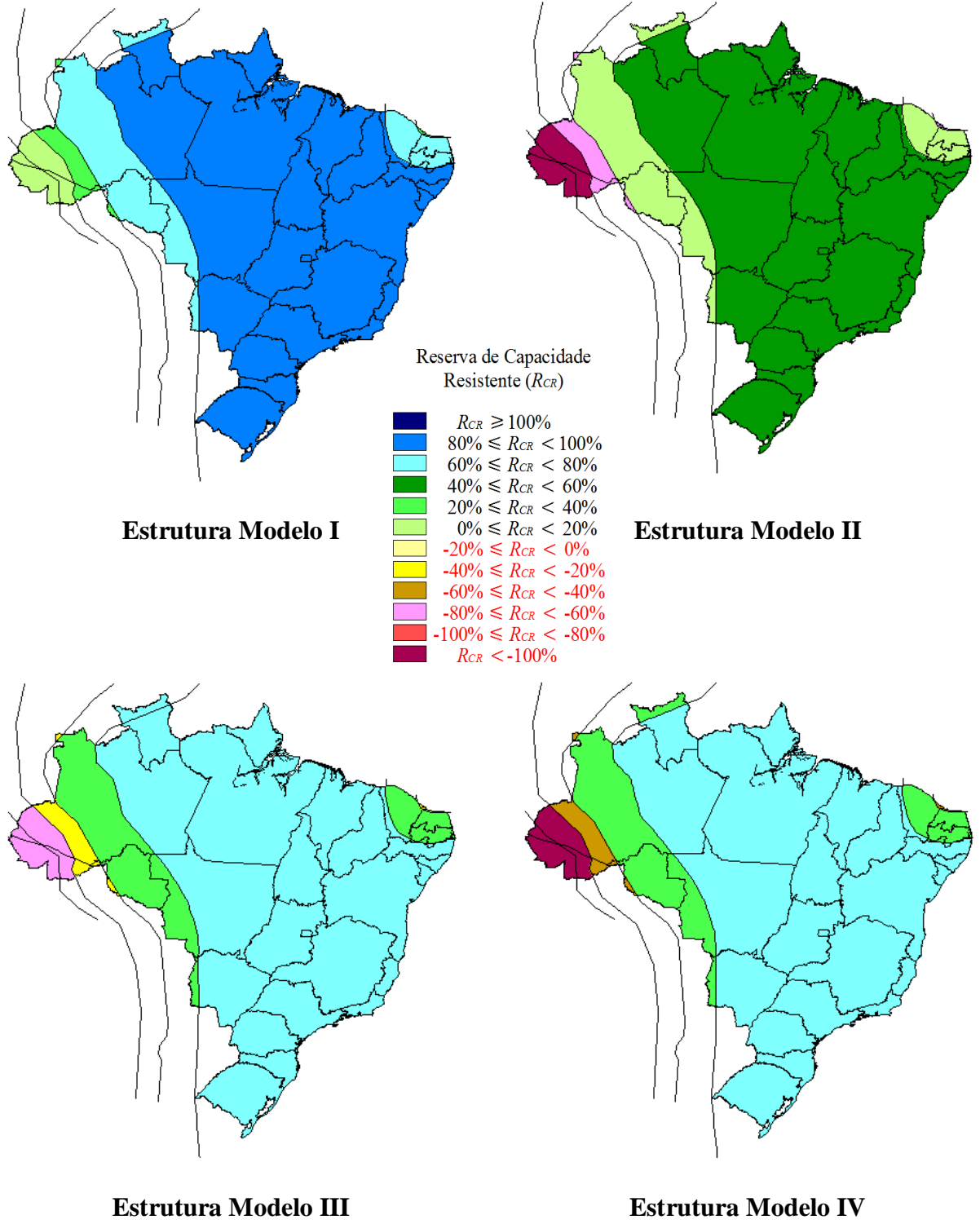
Figura 52 - Mapas de vulnerabilidade sísmica das estruturas modelo – Terreno Classe D
